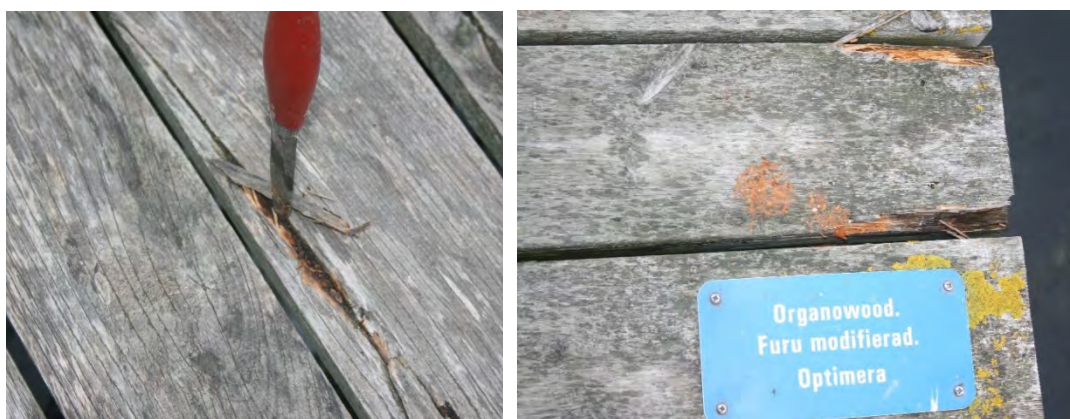
Figur 13. Rötangrepp i Organowood-modifierade plankor.
